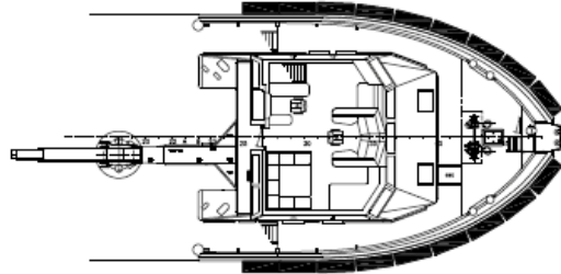
Maindeck
